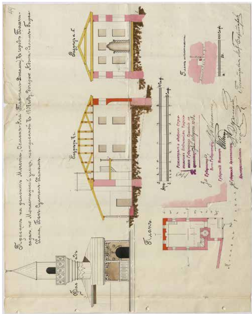
Рис. 1. «Проект на ремонт мечети Осман-Ага (Тахталы-Джами) в городе Бахчисарай по Монастырской улице...». Утвержден 2 августа 1913 г. [ГАРК, ф. 27, оп. 13, д. 4704, л. 44]
