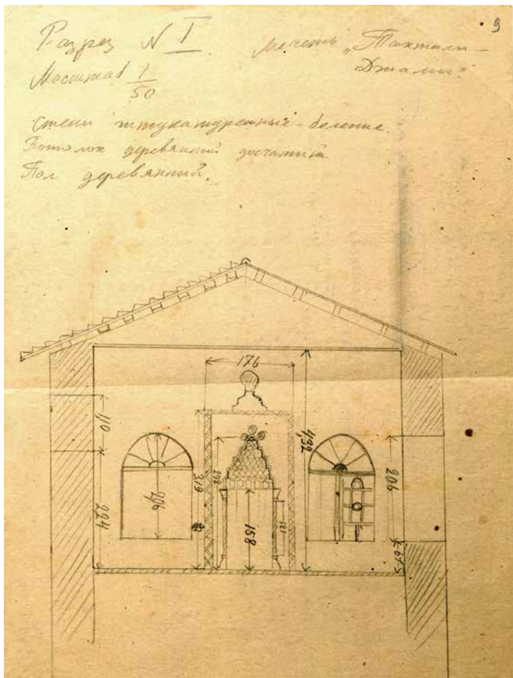
Рис. 7. «Разрез № 1. Мечеть Тахталы-Джами. Масштаб 1/50». Автор – А. Л. Ротач [ЦГАЛИ СПб, ф. Р-598, оп. 1, д. 169, л. 9]
