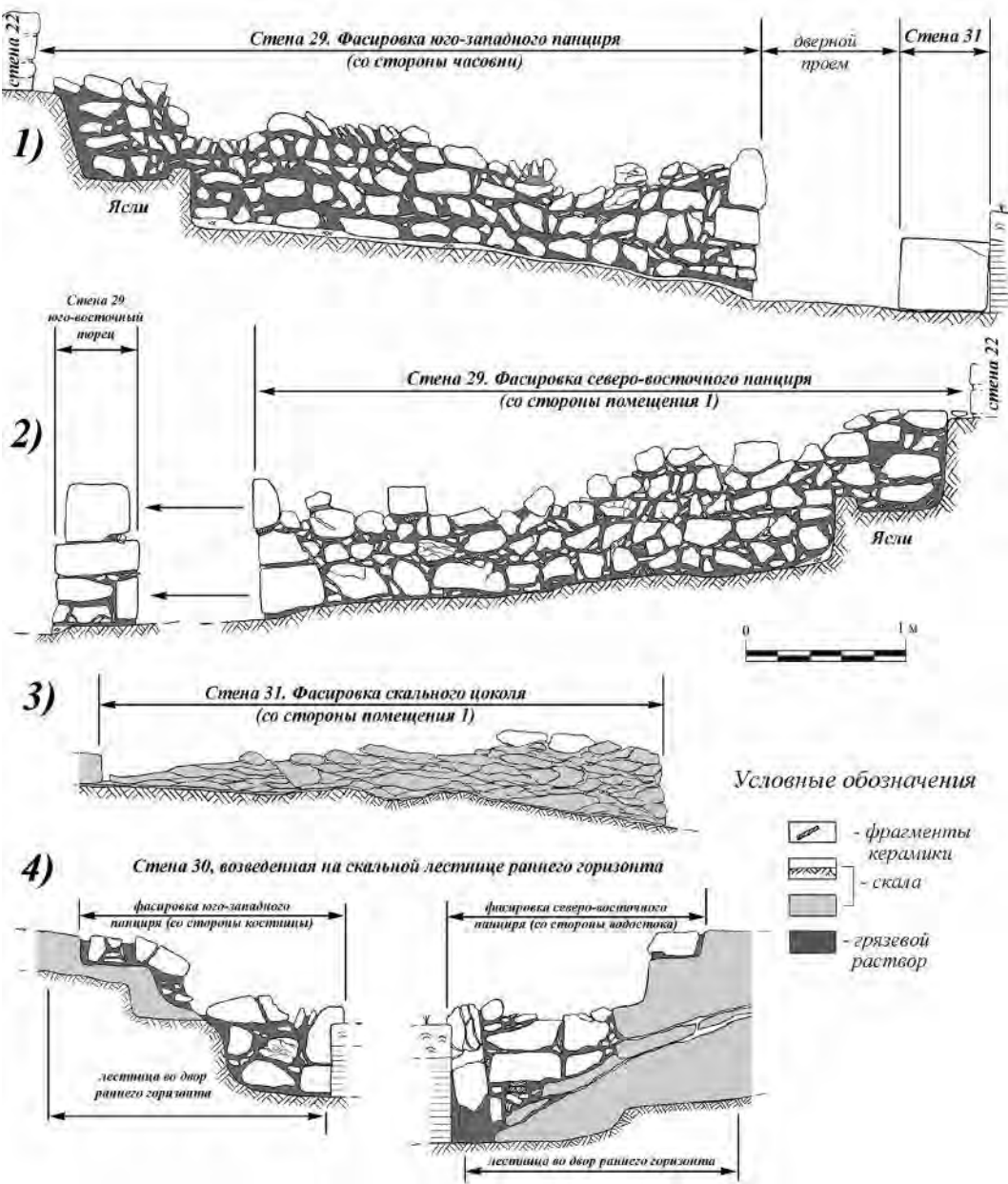
Рис. 6. Фасировки стен 29–30.
