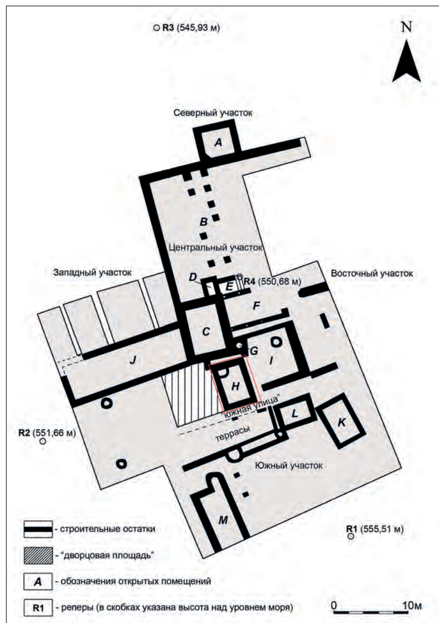
Рис. 2. Дворец. Общий план участков исследований 1912-1914, 1938, 1968, 1974 и 2006-2016 гг. (красным цветом выделено помещение H)
