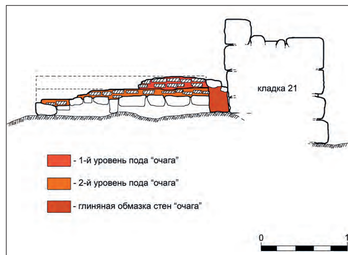
Рис. 10. Дворец. «Очаг» в северо-восточном углу помещения Н. Архитектурный разрез
