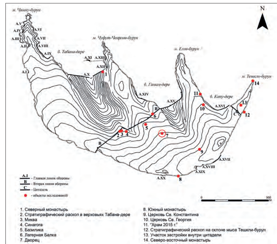
Рис. 1. Общий план Мангупского плато с указанием основных объектов археологических исследований в 1853-2016 гг.
