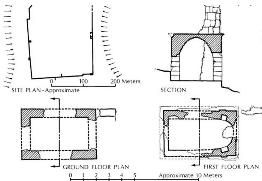
Рис. 5. План Сирменского монастыря с указанием места ворот, план северных ворот, план по уровню северной надвратной церкви, поперечный разрез северных ворот и храма [по: 14, fig. 115].
