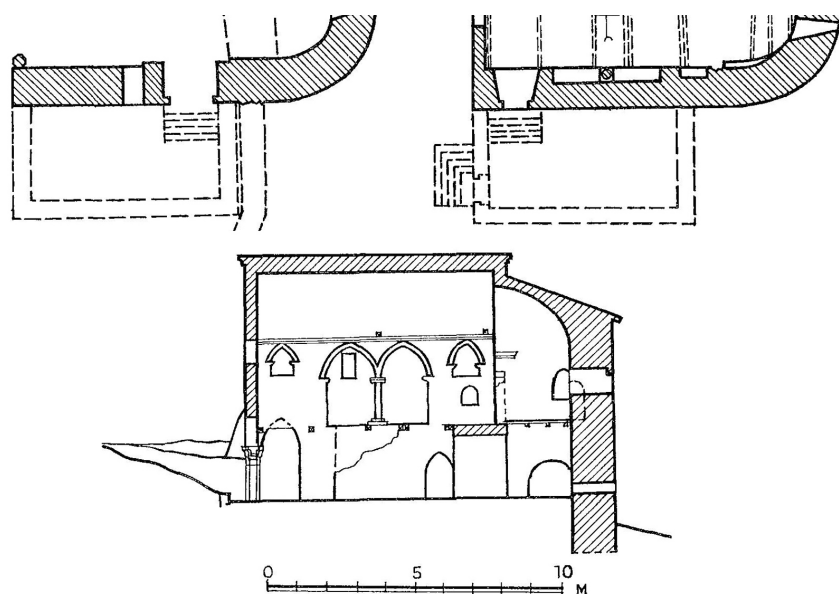
Рис. 7. План ворот и план и разрез надвратного храма в крепости Фуна [по: 3, рис. 9,9; 10,1].
