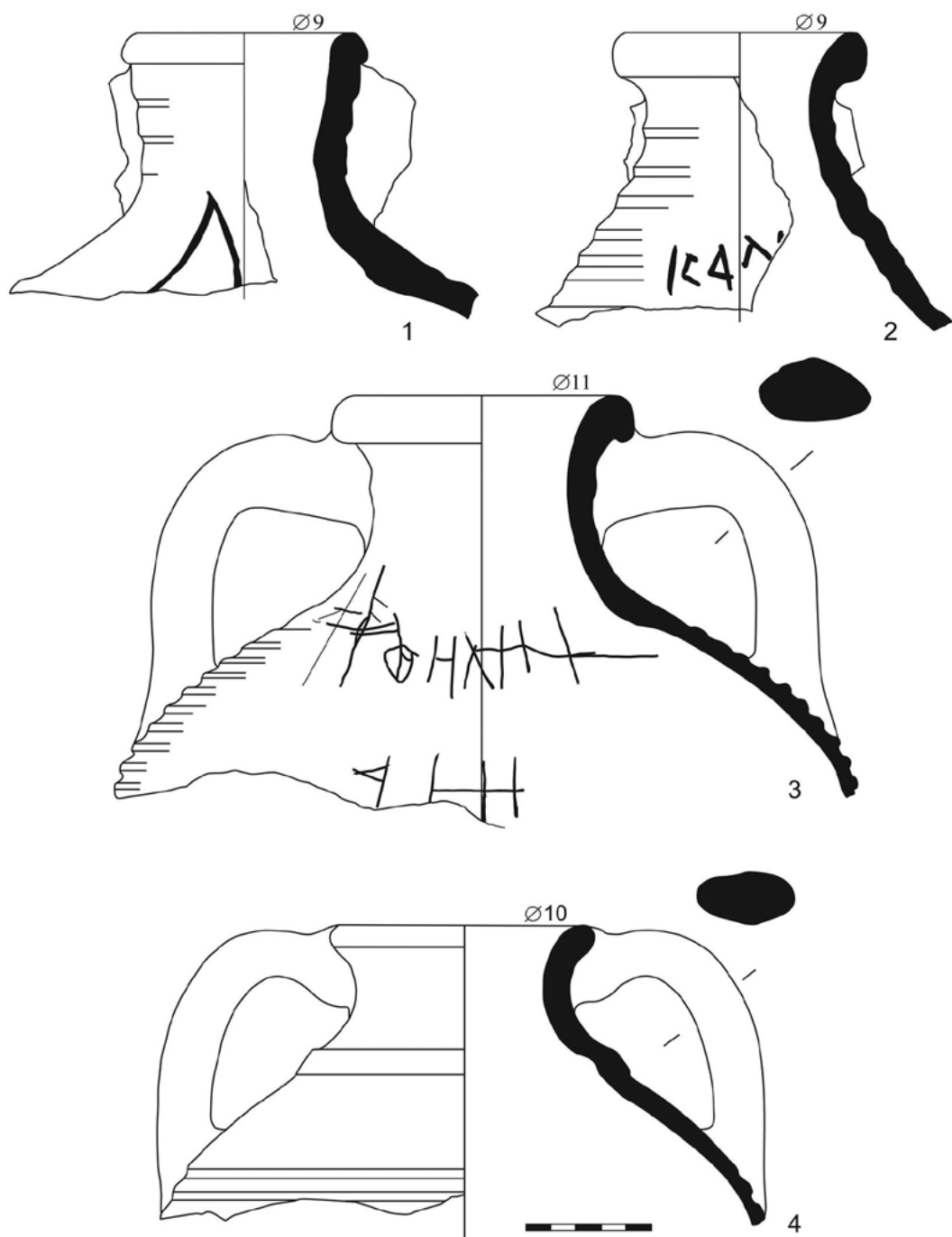
Рис. 3. Амфоры типа «Günşenin I» Fig. 3. Günşenin I amphorae
